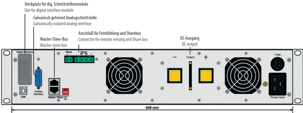
Rückansicht Standardmodell
